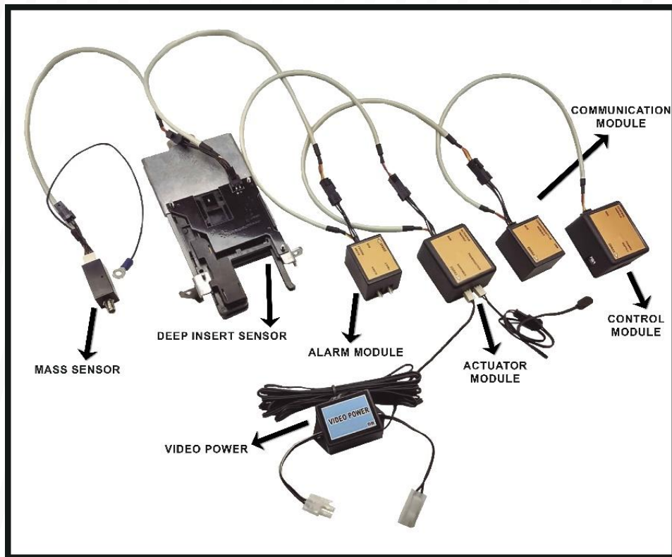
Figura 3 - Dispositivo Anti-Skimming Ebrax M.A.S.S.
