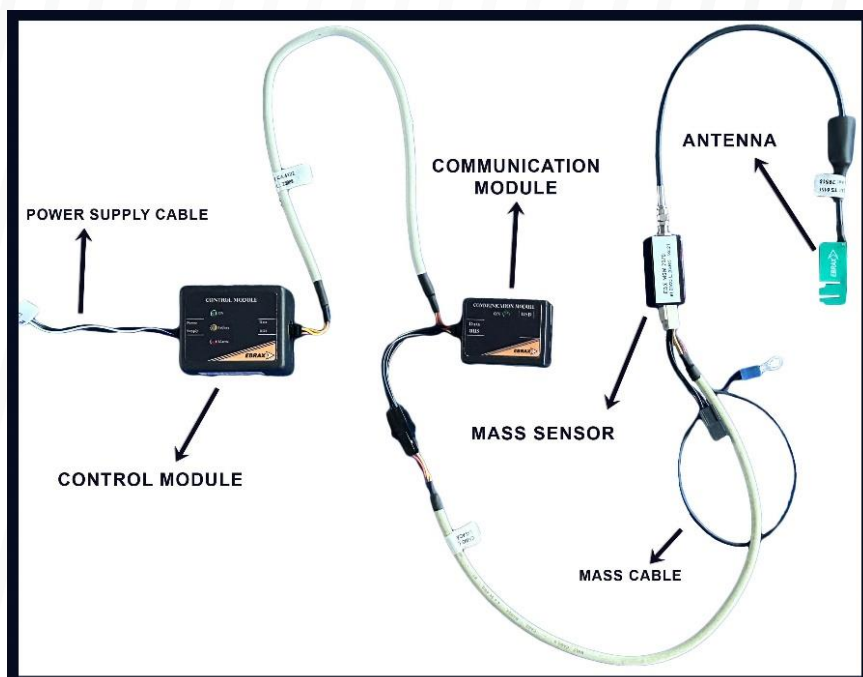
Figura 2 - Dispositivo Ebrax PS Anti-Skimming
