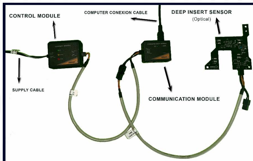
Figura 1 - Dispositivo Ebrax Anti-Shimming
